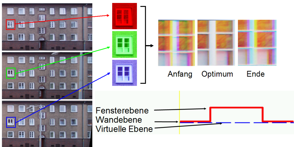
Abbildung 7.20: Planesweeping demonstriert an drei Bildern. Die Helligkeitswerte der drei Bilder wurden für eine gute Visualisierung den drei Farbkanälen Rot, Grün und Blau zugeordnet. Unterschiede zeigen sich damit in Form von Farben.
