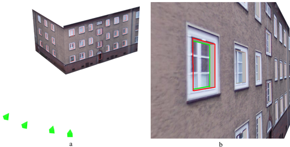
Abbildung 7.22: a) Fensterumrisse für zwei Fassaden als rote Rechtecke, 3D Fensterpositionen als grüne Rechtecke und Kamerapositionen als grüne Pyramiden; b) Detail für eine Fassade.
