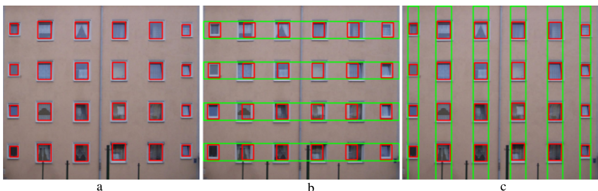
Abbildung 7.13: Modellauswahl – Repräsentation der Fassade durch a) Einzelfenster; b) Fensterzeilen; c) -spalten. Letztere bestehen aus Fenstern gleicher Größe mit konstantem horizontalen bzw. vertikalen Abstand.
