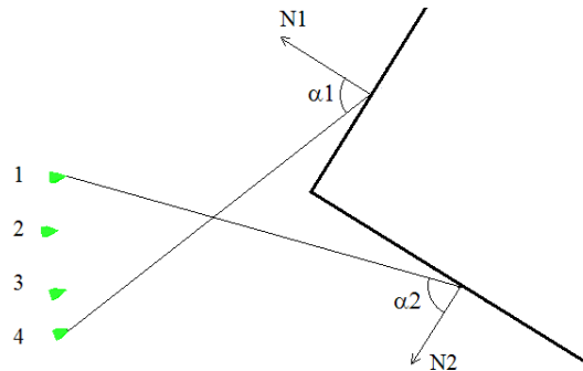
Abbildung 7.21: Winkel zwischen Verbindungslinien von Kameraposition und Fassadenmitte zu den Normalen der Fassadenebenen N1 und N2 . Die Kamerapositionen sind als grüne Pyramiden dargestellt.
