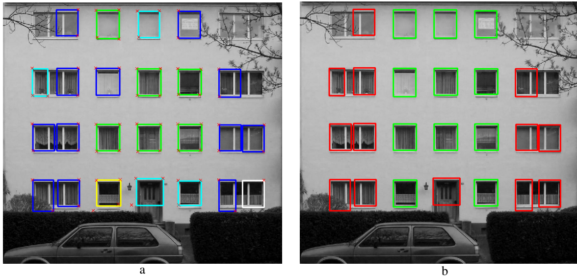
Abbildung 7.12: Fenstererkennung: a) Vor der Validierung. Rote Kreuze – Erkannte Ecken, Grüne Rechtecke – Sehr gut, Gelb – Gut, Cyan – Ausreichend, Blau – Schlecht; b) Nach der Validierung. Grüne Rechtecke – akzeptierte Objekte, rote Rechtecke – abgelehnte Objekte. Breite Fenster sind nicht im Trainingsdatensatz enthalten und werden deswegen nicht korrekt erkannt.
