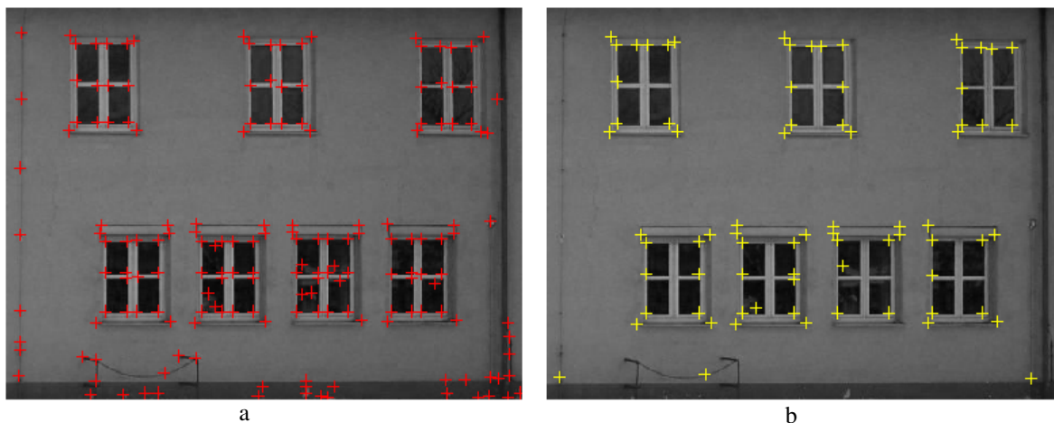
Abbildung 5.7: Extrahierte Förstnerpunkte; b) akzeptierte Förstnerpunkte.
