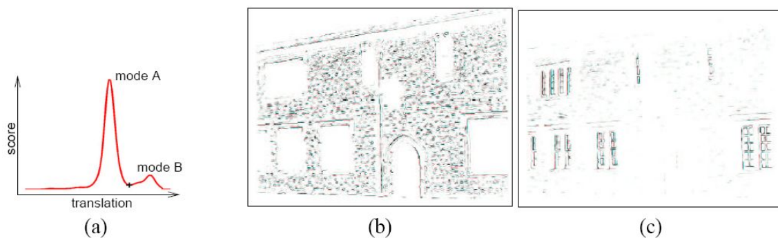
Abbildung 3.8: (a) Bewertung der Ähnlichkeit der drei gegebenen Ansichten bei Translation der virtuelle Ebene senkrecht zur Fassade. Mode A entspricht der Fassadenebene und Mode B der Fensterebene. Die Ähnlichkeiten für Punkte auf der Fassade sind in (b) für den Mode A und in (c) für den Mode B dargestellt (WERNER UND ZISSERMAN 2002).
