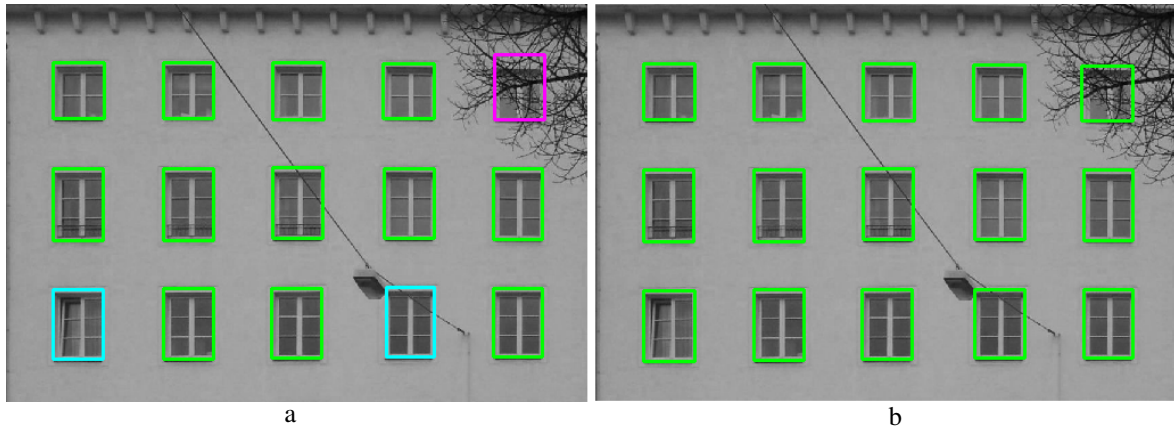
Abbildung 7.10: a) Ergebnis vor der Validierung der Objekte; b) Endgültiges Ergebnis.
