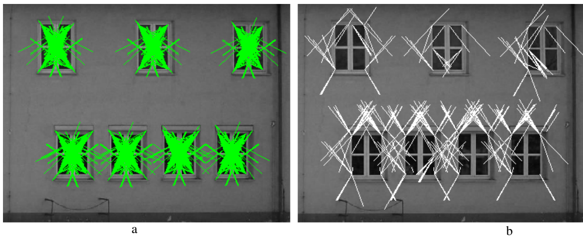
Abbildung 7.1: Filterung der Zuordnung von Bild- und Trainingsausschnitten: a) Akzeptierte Differenzvektoren; b) Abgelehnte Differenzvektoren.
