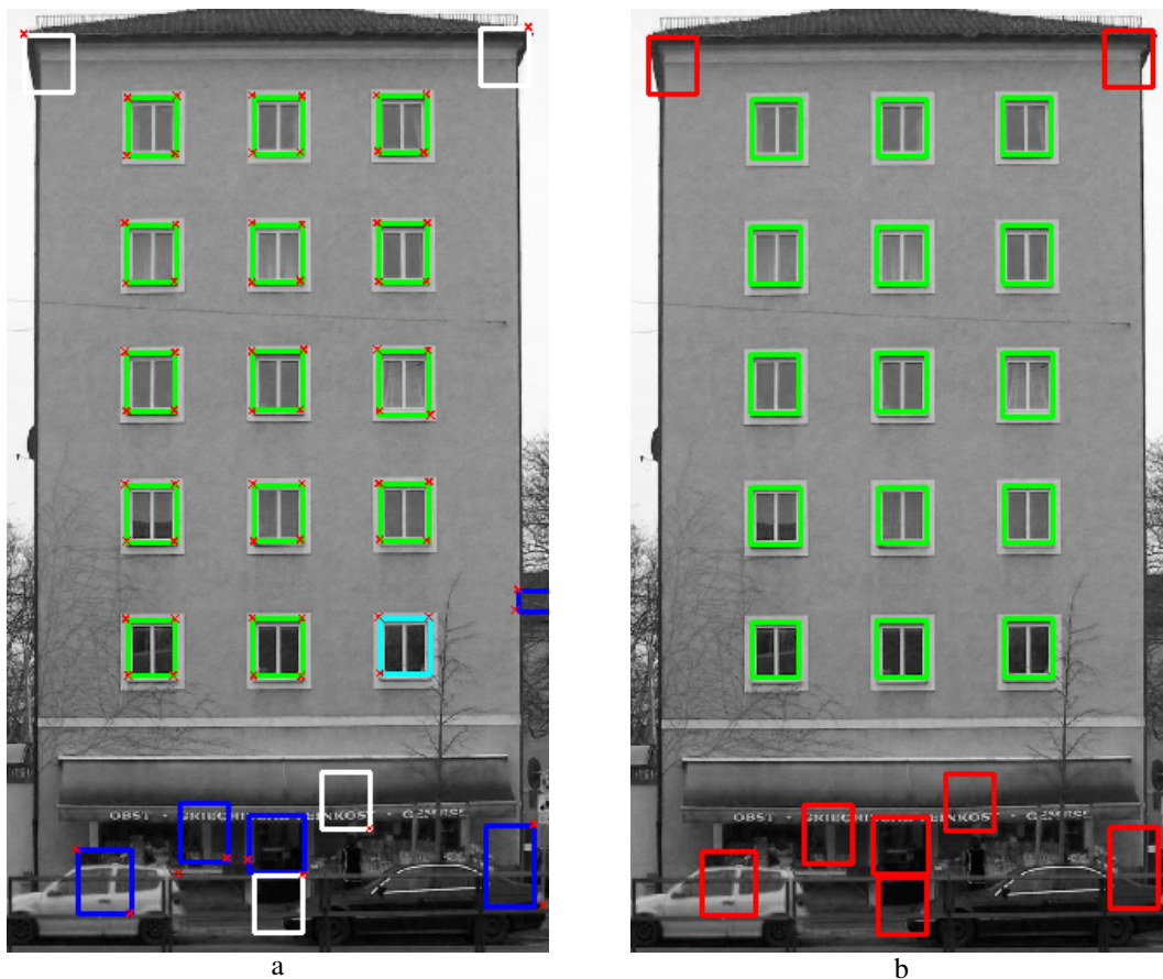
Abbildung 7.6: Fenstererkennung: a) Vor der Validierung. Rote Kreuze – Erkannte Ecken, Grüne Rechtecke – Sehr gut, Hellblaue – Ausreichend, Blau – Schlecht, Weiß – Sehr schlecht; b) Nach der Validierung. Grüne Rechtecke – akzeptierte Objekte, rote Rechtecke – abgelehnte Objekte.
