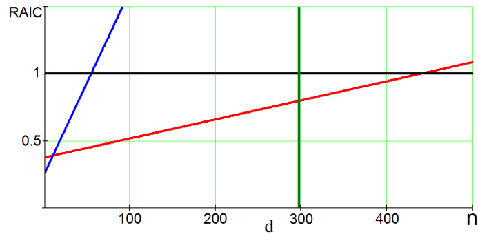
Abbildung 8.1: Ergebnis der Optimierung mittels MCMC a) Einzelfenstermodell, Anzahl Parameter für Modell k = 96 ; b) Spaltenmodell, k = 36 ; c) Zeilenmodell, k = 24 . d) Abhängigkeit RAIC von n (Einzelfenster – schwarz, Spalten – rot, Reihen – blau, minimale Umrisslänge – grün)
