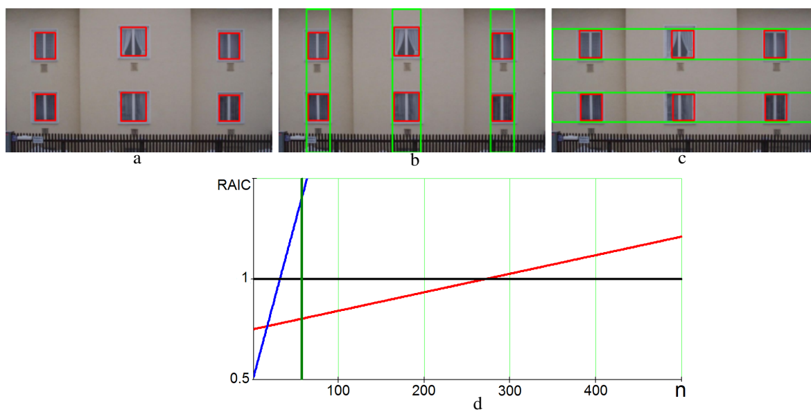
Abbildung 8.3: Ergebnis der Optimierung mittels MCMC a) Einzelfenstermodell, k = 24 ; b) Spaltenmodell, k = 18 ; c) Zeilenmodell, Anzahl von Parameter für Modell k = 12 . d) Abhängigkeit RAIC von n (Farben siehe Abbildung 8.1)
