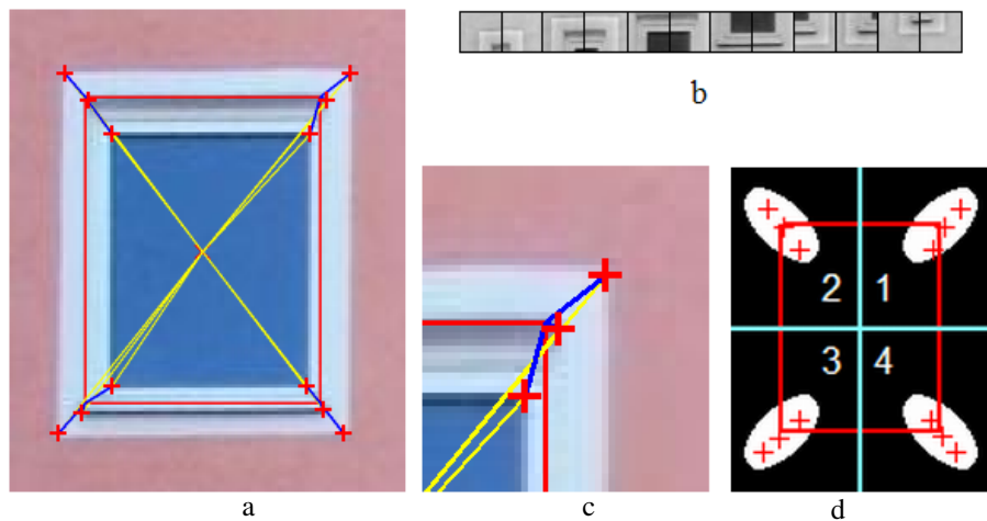
Abbildung 5.4: Training für Fensterdetektion und Segmentierung - a) Bildausschnitt mit manuell vorgegebenem Fensterumriss (rotes Rechteck), Förstnerpunkte an den Ecken des Fensterumrisses (rote Kreuze) sowie Vektoren von den Förstnerpunkten zum Fenstermittelpunkt (gelbe Linien) und zu der korrespondierenden Ecke des Umrisses (kurze blaue Linien); b) Bildausschnitte um die Förstnerpunkte; c) Detail von a) zeigt das Verhältnis der Förstnerpunkte zu einer Ecke des Fensters; d) Elliptische Flächen um die Fensterecken (weiß) in denen die Förstnerpunkte extrahiert werden.
