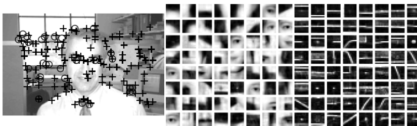
Abbildung 2.1: Förstner Interest Punkte in einem Trainingsbild eines menschlichen Gesichtes mit verrauschtem Hintergrund (links). Kreuze kennzeichnen eckige Muster während Kreise runde Muster markieren. In der Mitte sind Cluster von Bildausschnitten für Gesicht und rechts für Autos, Letztere in Form der Gradienten, dargestellt. (WEBER et al. 2000).
