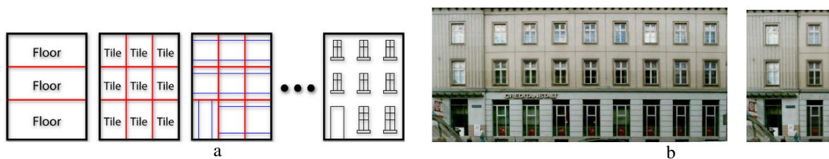
Abbildung 3.5: a) – Hierarchische Unterteilung der Fassade. b) – Links: die Fassade aus Abbildung 3.4 nach der Entfernung der senkrechten Symmetrie. Rechts: Die Beseitigung der horizontalen Symmetrie resultiert in einer nicht reduzierbaren Fassade (VAN GOOL et al. 2007).
