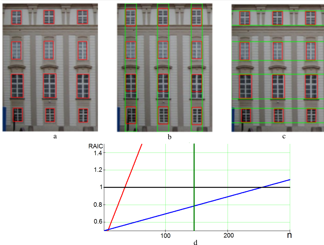
Abbildung 8.2: Ergebnis der Optimierung mittels MCMC a) Einzelfenstermodell, k = 48 ; b) Spaltenmodell, k = 18 ; c) Zeilenmodell, Anzahl von Parameter für Modell k = 24 . d) Abhängigkeit RAIC von n (Farben siehe Abbildung 8.1)
