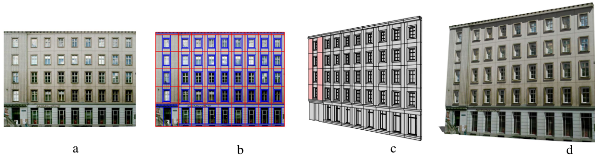
Abbildung 3.4: Mittels der grammatikbasierten Rekonstruktion können Fassadentexturen in ein semantisches 3D Modell hoher Qualität konvertiert werden. a) – Orthogonalisiertes Fassadenbild als Eingabe; b) – Automatisch unterteilte Fassade; c) – Polygonales 3D Modell als Ergebnis; d) – Visualisierung mit Schatten und Spiegelungen (VAN GOOL et al. 2007).
