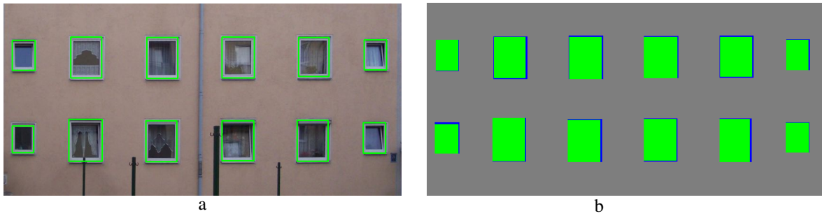
Abbildung 8.11: Ergebnisse für Fassade 1: a) Segmentierung durch ISM (grüne Rechtecke); b) Evaluierung (Farben siehe Abbildung 8.9)
