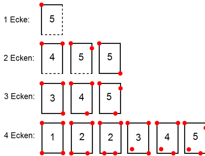
Abbildung 7.4: Notensystem für rechteckige Objekte – eine bessere Note bedeutet eine höhere Verlässlichkeit. Für symmetrische Konfigurationen ist jeweils nur eine Möglichkeit angegeben.
