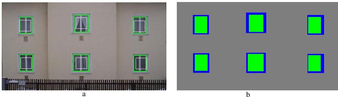
Abbildung 8.10: Ergebnisse für Fassade 2: a) Start von MCMC (weiße Rechtecke) und Endergebnis (grüne Rechtecke); b) Evaluierung (Farben siehe Abbildung 8.9)
