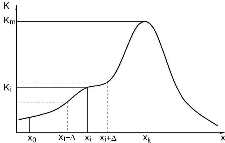
Abbildung 2.6: Der Entscheidungsprozess für eine eindimensionale Markovkette.
