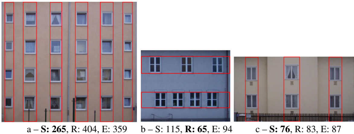
Abbildung 7.15: Modellauswahl unter Verwendung von AIC – S: Spalten, R: Reihen, E: Einzelfenster; gewählte Modelle sind fett dargestellt.
