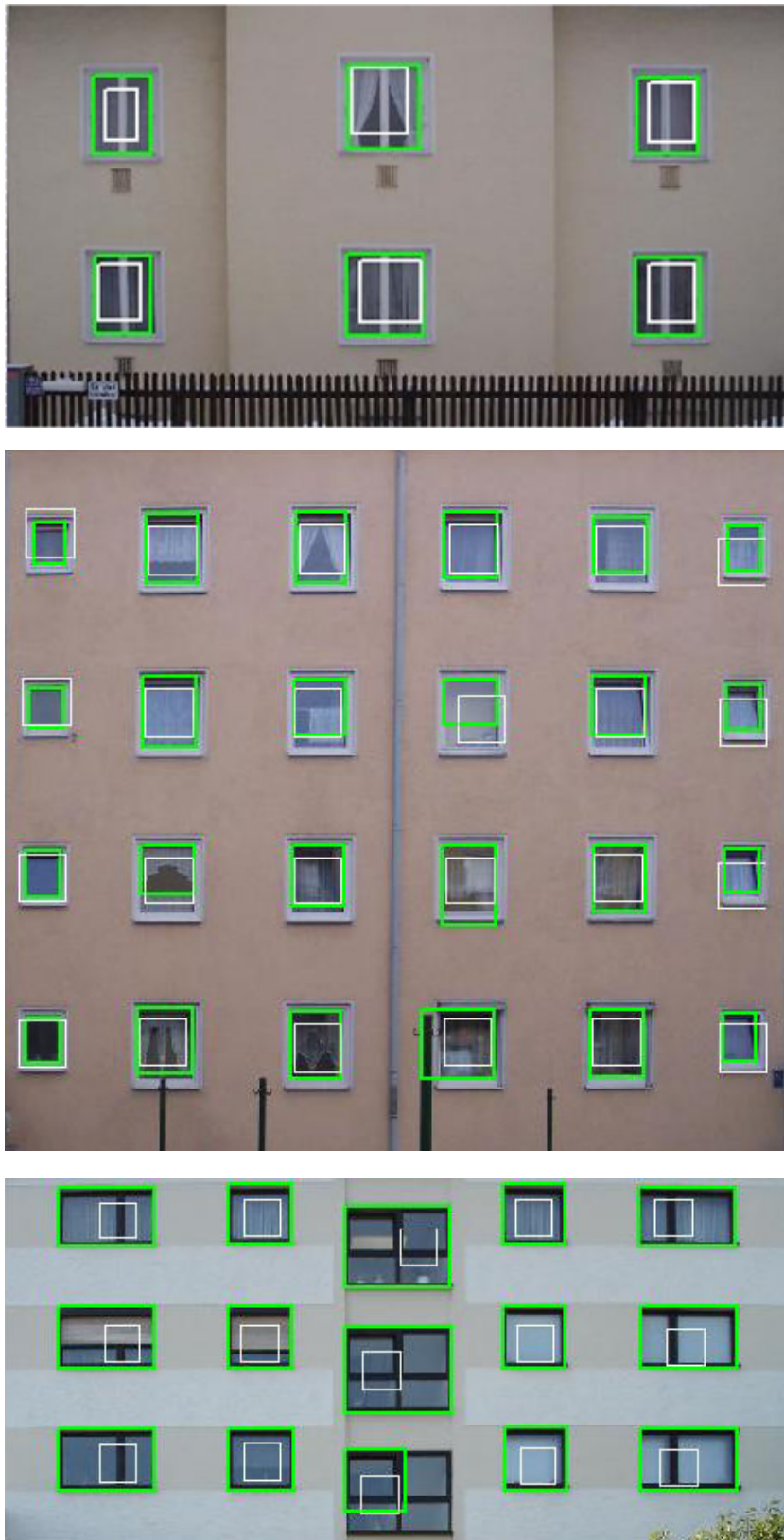
Abbildung 6.4: Weitere Ergebnisse für dunkle Fenster auf hellen Fassaden – Hypothesen (weiße Quadrate) und Fenster (grüne Rechtecke).
