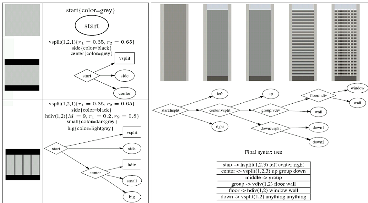
Abbildung 3.3: Modellierung der Bestandteilshierarchie für eine Fassade mittels einer stochastischen kontextfreien Grammatik (ALEGRE und DALLAERT 2004).
