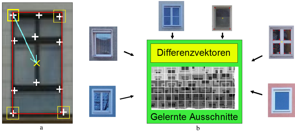
Abbildung 5.3: a) – Fenster mit manuell markiertem Umriss (rotes Rechteck), Förstnerpunkte (weiße Kreuze) und ein Differenzvektor eines Förstnerpunktes in der Nähe einer Fensterecke zur Fenstermitte (blauer Pfeil); b) – Gelernte Differenzvektoren und Bildausschnitte um Förstnerpunkte für eine Fenstermenge (Trainingsdatensatz).
