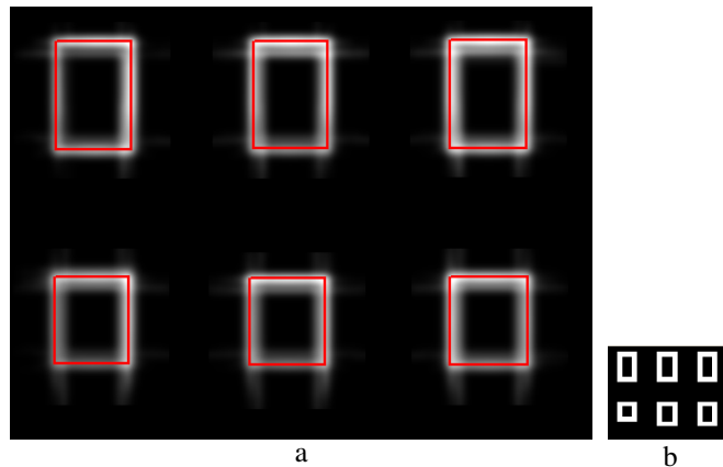
Abbildung 7.14: Definition von Likelihood für den Fensterumriss – a) Verteilungsbild mit Fensterumrissen als rote Rechtecke; b) Auf minimale Größe reduziertes Verteilungsbild.
