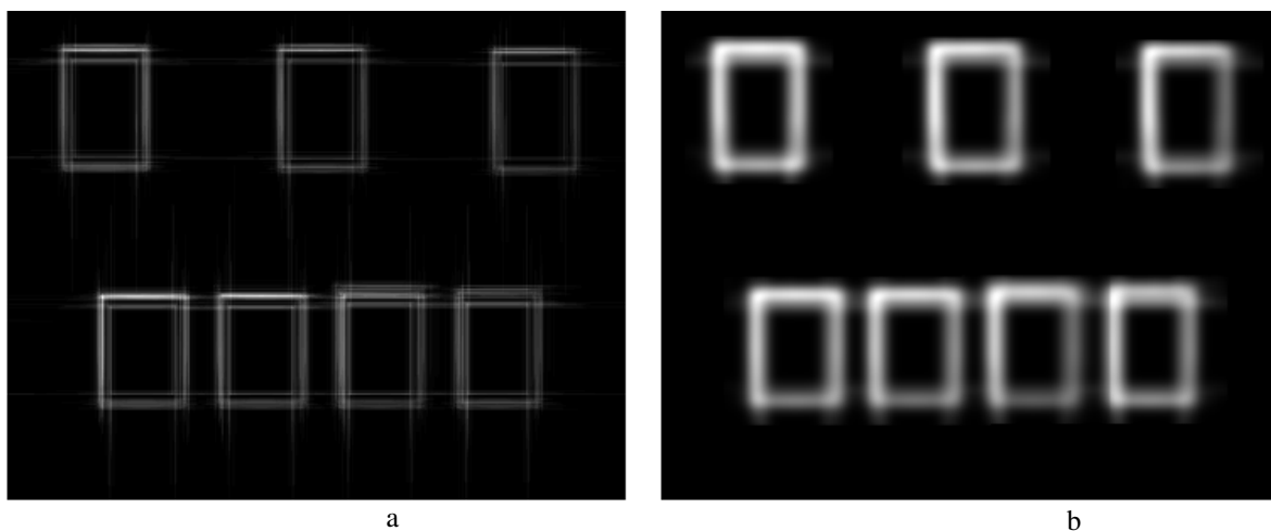
Abbildung 7.3: a) Verteilung für Fensterumrisse auf ganzer Fassade – a) Akkumulation; b) Nach Glättung und Normalisierung.
