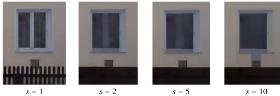
Abbildung 2.5: Morphologischer Maßstabsraum.
