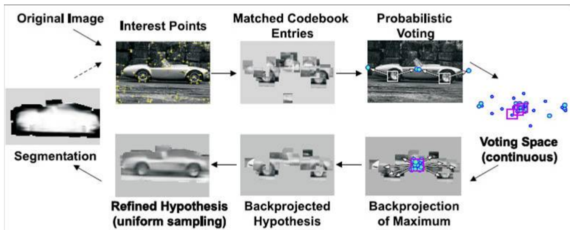
Abbildung 2.3: Implicit Shape Models . (LEIBE und SCHIELE 2004b)
