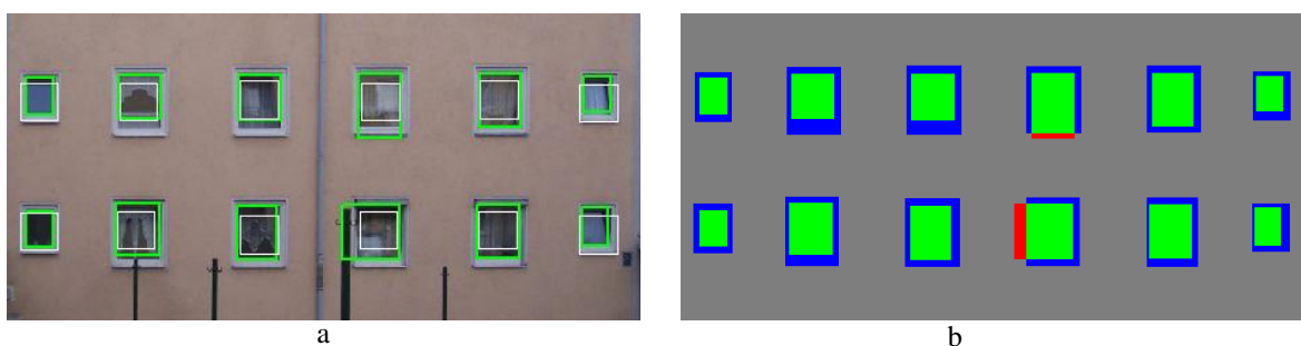
Abbildung 8.9: Ergebnisse für Fassade 1: a) Start von MCMC (weiße Rechtecke) und Endergebnis (grüne Rechtecke); b) Evaluierung (korrekt – grün, Referenz – blau, inkorrekt – rot)
