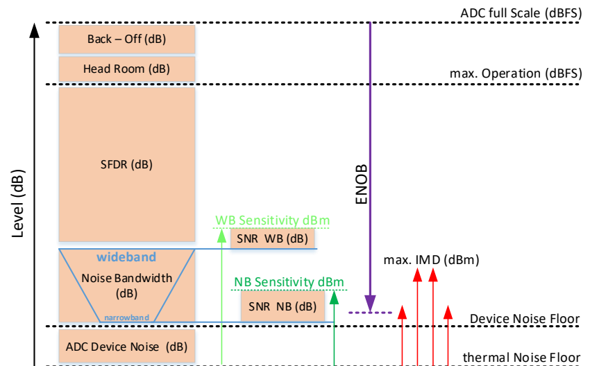
Δ Fig. 4 ADC parameters at a glance
