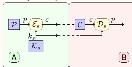
Abbildung 3.1.: Symmetrische Chiffrierung
