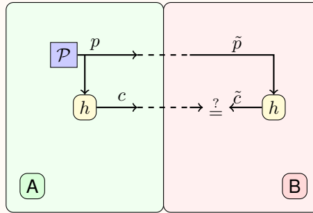
Abbildung 8.1.: Hashwert-Erzeugung
