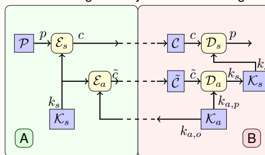
Abbildung 6.2.: Hybride Chiffrierung
