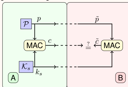
Abbildung 8.2.: Message Authentication Code-Erzeugung
