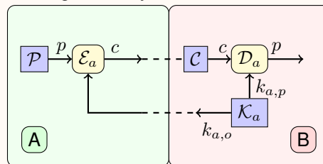
Abbildung 6.1.: Asymmetrische Chiffrierung
